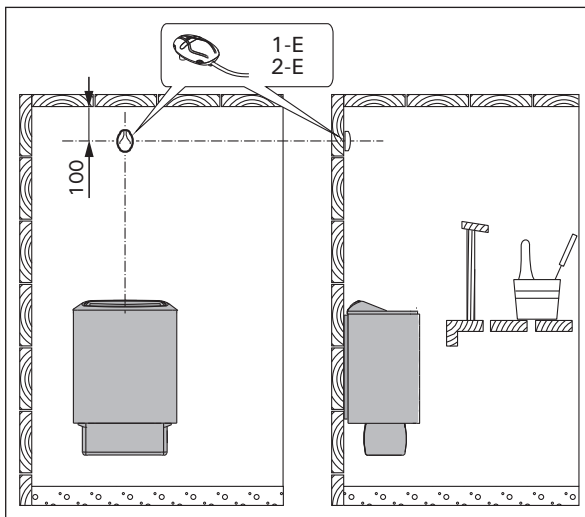
Figure 11. Installation du capteur (toutes les dimensions sont fournies en millimètres) Figuur 11. De sensor installeren (alle afmetingen in millimeters)
