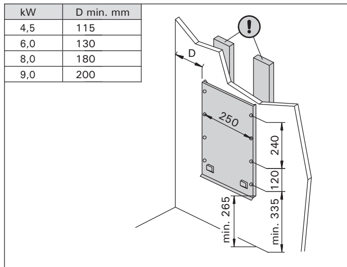
9. ábra A fali szerelvény elhelyezése (a méretek milliméterben értendők) Bild 9. Placering av aggregatets monteringsställning (måtten i millimeter)
