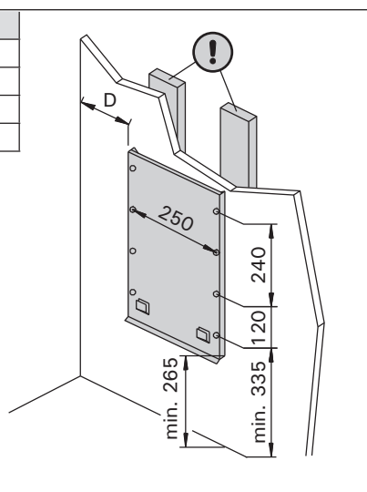
Rys. 9. Lokalizacja wieszaka monta¿owego pieca (wymiary w milimetrach) Obrázek 9. Umístění montážní konzoly na kamnech (všechny rozměry jsou v milimetrech)
