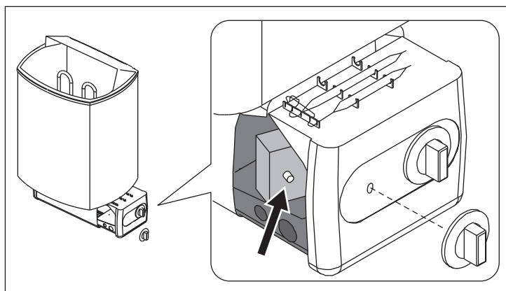
Rys. 12. Przycisk resetowania wy³ącznika termicznego (1) Obrazek 12. Resetovací tlačítko ochrany proti přehřátí (1)
