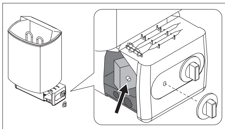
Figura 12. Botão de reposição do protetor de sobreaquecimento (1)
