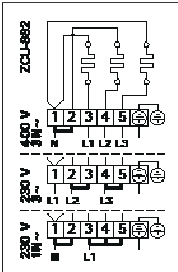
Rys. 14. Schemat elektryczny (1-E, 2-E) Obrazek 14. Zapojení topného tělesa 1-E, 2-E
