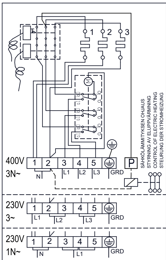
Rys. 13. Schemat elektryczny (1) Obrazek 13. Zapojení topného tělesa 1
