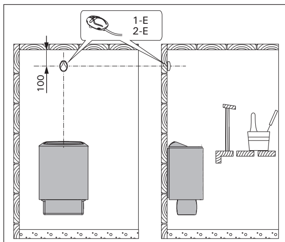
Rys. 11. Instalowanie czujników (wymiar w milimetrach) Obrazek 11. Instalace snímače (všechny rozměry jsou v milimetrech)
